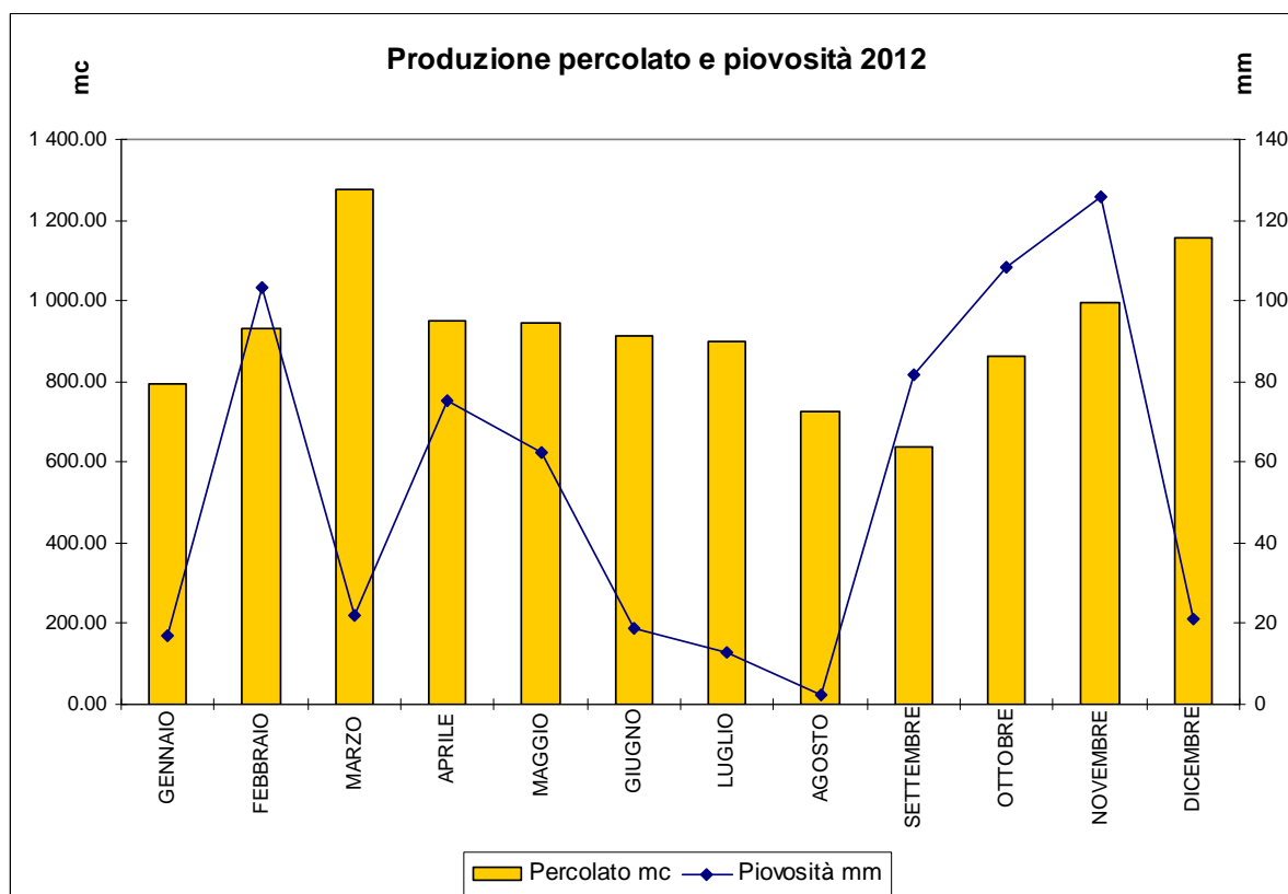
Grafico n. 1 – Andamento della produzione di percolato e piovosità in discarica Rio Riazzone nell'anno 2012
