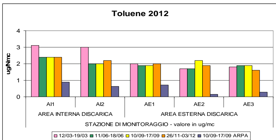
Grafico n. 3 – Andamento Toluene, anno 2012
