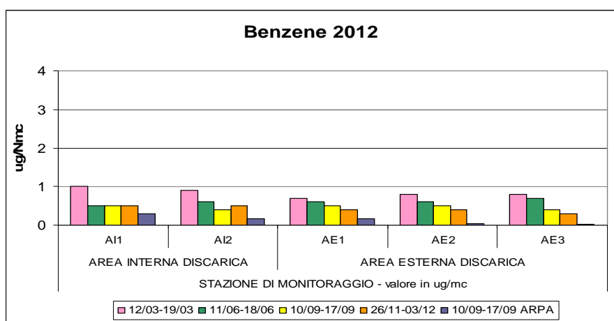
Grafico n. 2 – Andamento Benzene, anno 2012
