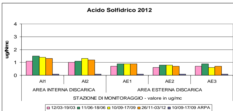
Grafico. n 5 – Andamento Acido Solfidrico, anno 2012
