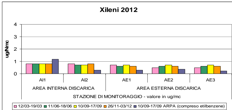
Grafico n. 4 – Andamento Xileni, anno 2012
