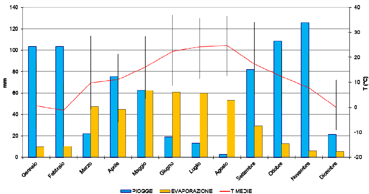
Grafico. n. 6 – Andamento di Temperature medie mensili, piovosità ed evapotraspirazione rilevati presso la Discarica di Rio Riazzone, anno 2012
